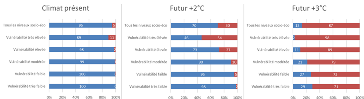
Figure 32 – Part de la population exposée à un aléa modéré à très élevé (en rouge) en fonction de leur vulnérabilité socio-économique selon le climat présent et des futurs à +2°C et +3°C.
