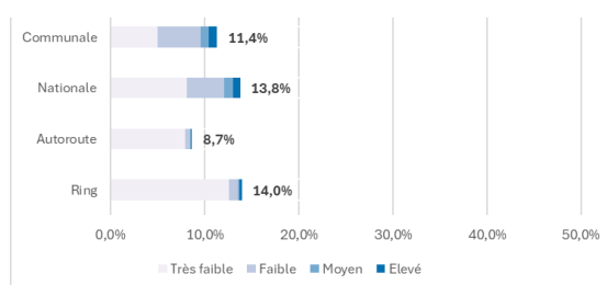
Figure 40 – Part des routes exposées aux inondations par type de route et niveau d'aléa.
