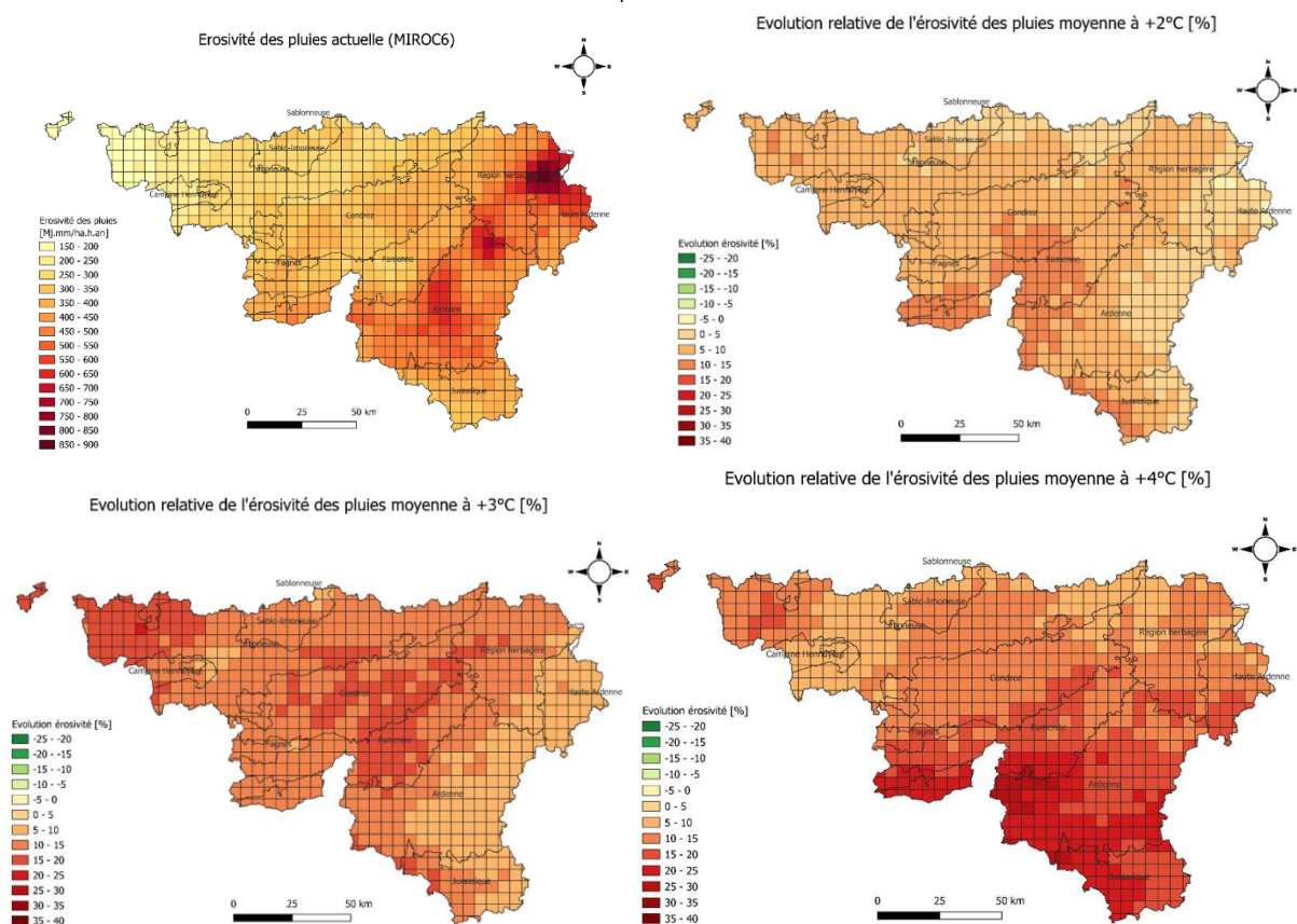
Figure 7 - Erosivité des pluies actuelle et évolution dans un monde à +2°, +3° et +4°C pour la moyenne des modèles globaux.
