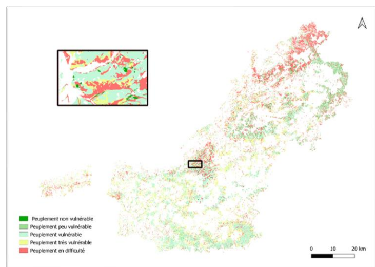
Figure 3 - carte de la vulnérabilité des peuplements purs de hêtres et d’épicéas en Ardenne dans un niveau de réchauffement global de +4°C.
