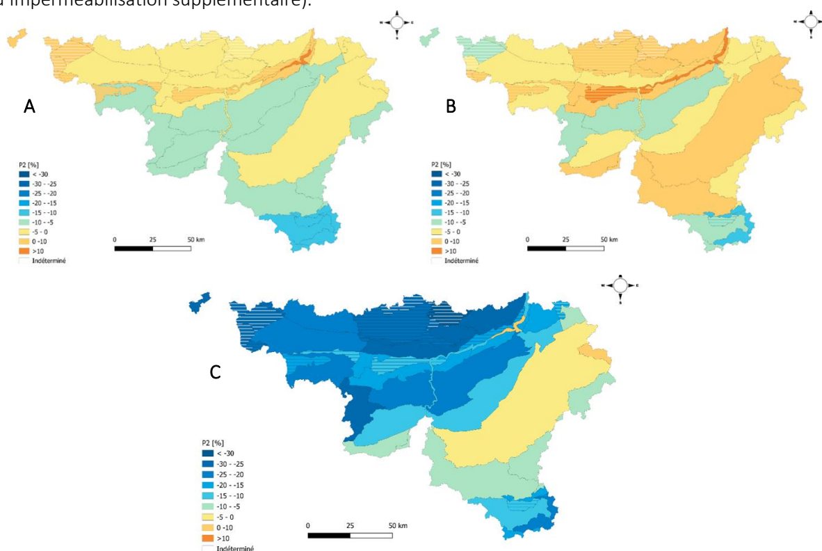
Figure 8 - Evolution du risque pour l'approvisionnement des nappes en pourcentage dans un monde à +2° (A), +3° (B) et +4°C (C) pour le modèle extrême sec CMCC.
